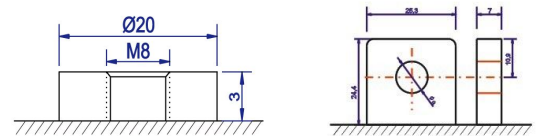
M8 Bolt
