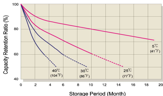
不同温度下的容量保存率特性
