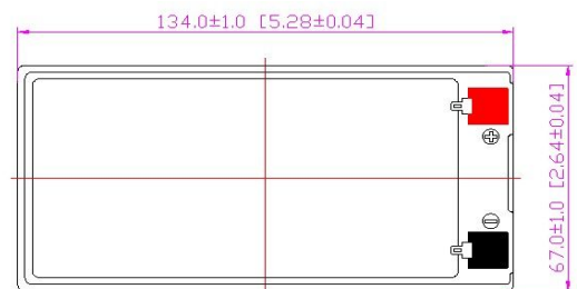
F1 Terminal
