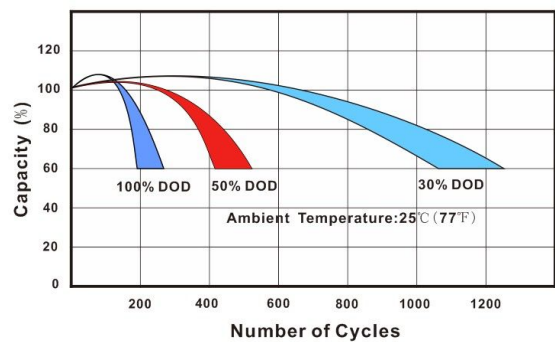
不同放电深度下的循环寿命特性
