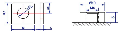
M5 Bolt & Nut T1 Terminal
